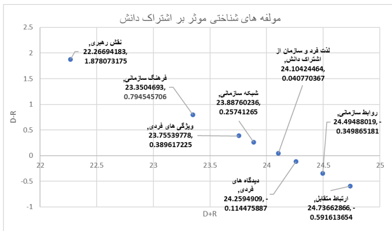
شکل ۷: ماتریس ((I-X)X.\text{INVERS})
